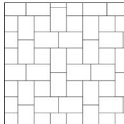
LA PIAZZA 3 Keresztkötes Kőigény (ca): TÉGLAKŐ 12,5 db/m 2 NÉGYZETKŐ 6,3 db/m 2
