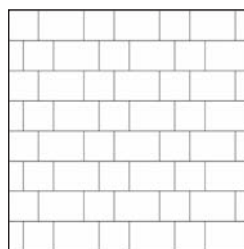
SUAVE 5 Gótikus kötés Kőigény (ca): 1 1/2 KŐ 15,63 db/m 2 NORMÁLKŐ 15,63 db/m 2
