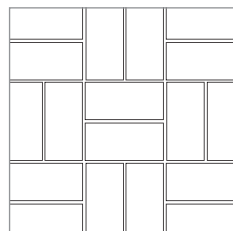
BETONTÉGLA 4 Sakktáblakötés Kőigény (ca): NORMALKŐ 32 db/m 2
